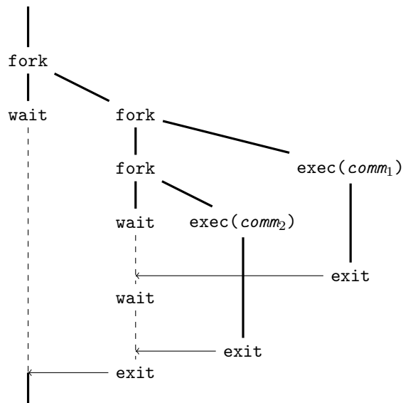
FIGURE 5.2 – Enchaînement parallèle de processus : comm_1 \mid comm_2
