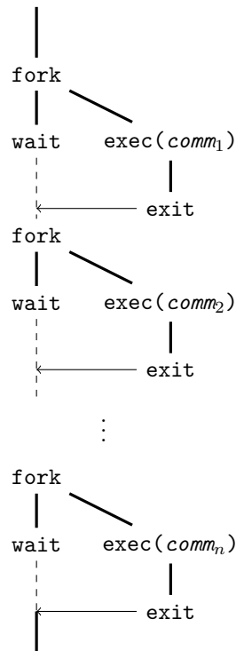
FIGURE 5.1 – Enchaînement séquentiel de processus
